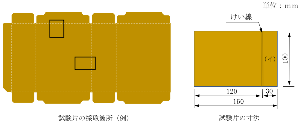
図2 試験片の採取場所 (例) と寸法
