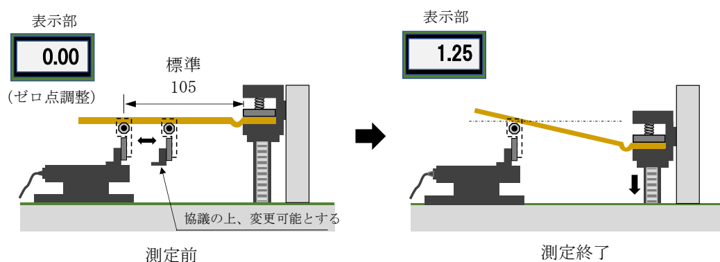
図3 操作 (試験)
